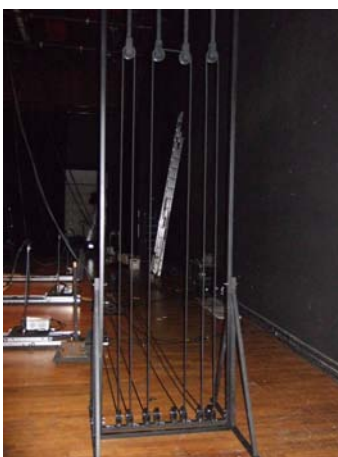
Lest (700kg) pour Trapèze (fenêtre)
